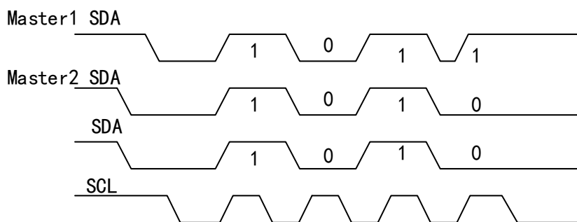
图 80 SDA 时序图
