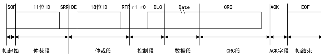
图 102 扩展数据帧
