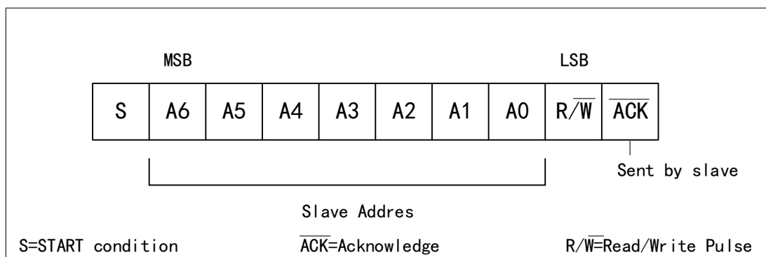
图 82 7 位地址格式
